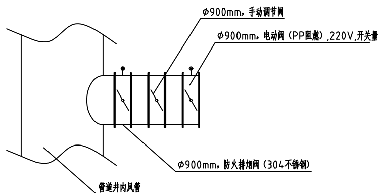
2#楼废气处理系统管道井风管支管接口大样图
