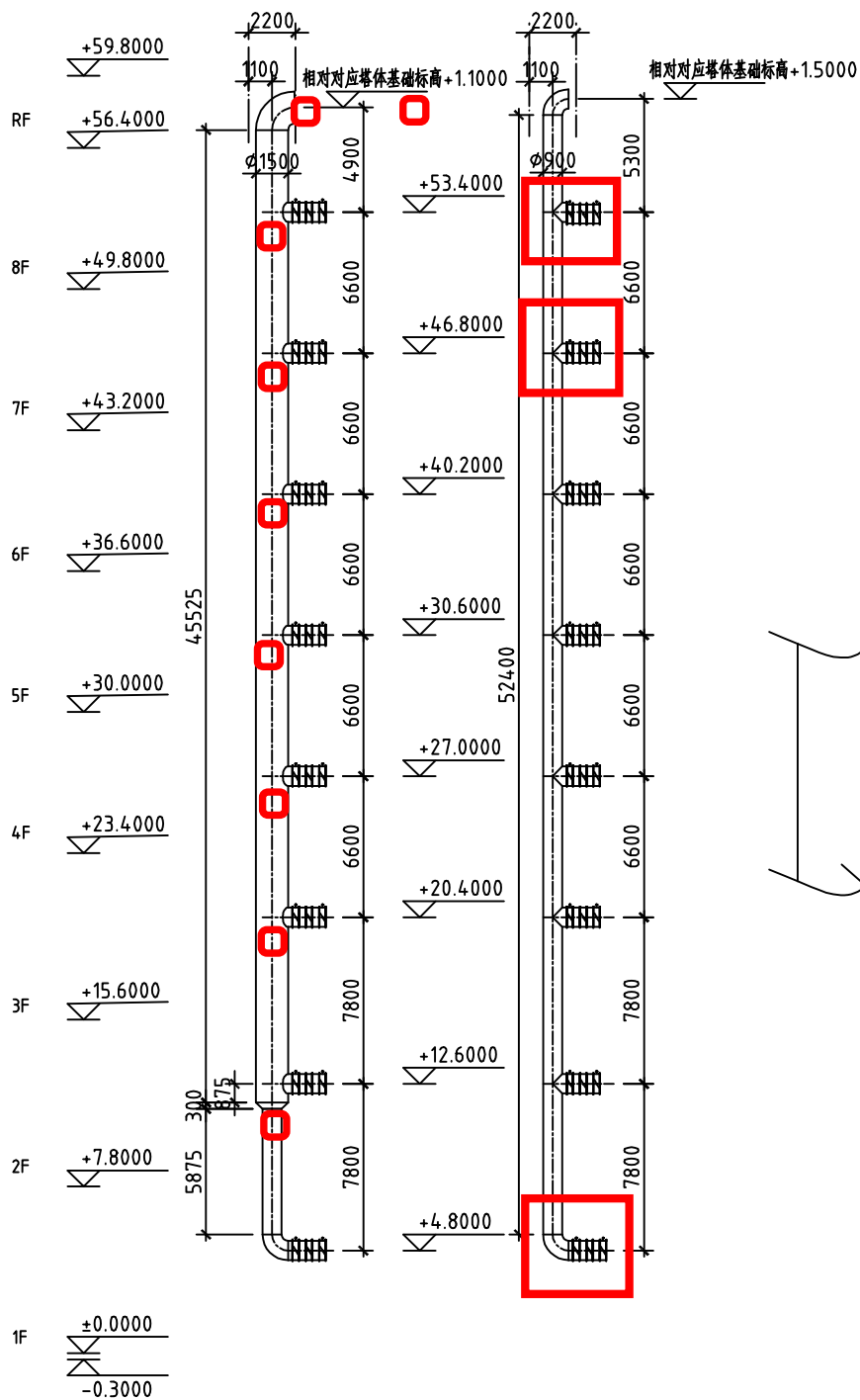
2#楼废气处理系统管道井风管支管接口大样图
