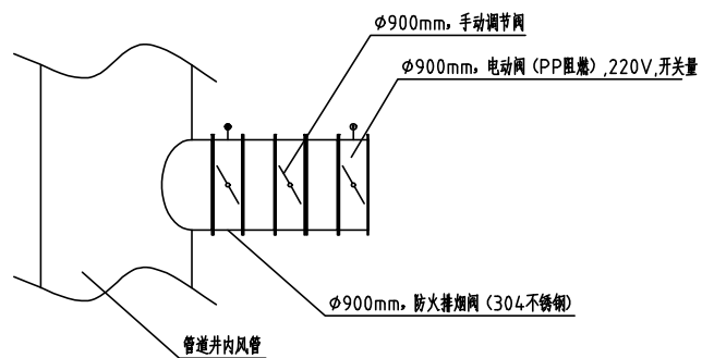
3#楼废气处理系统管道井风管支管接口大样图
